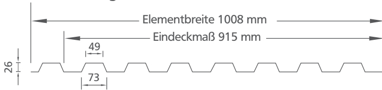
Profilgeometrie - MSL-TRAPEZPROFIL
