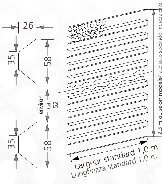
Tôle perforée à profilage trapézoïdal 58-35 /26 mm Lamiera perforata con nervatura a profilo trapezoidale 58-35 /26 mm
